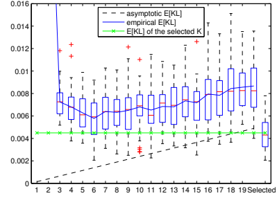
(d) Example MS with 10 000 data points
